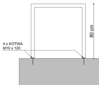
STOJAK MODERN 2 MK MONTAŻ KOTWY
