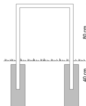
STOJAK MODERN 2 MB MONTAŻ BETON
