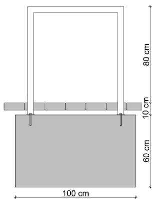
STOJAK MODERN 2 MKB MONTAŻ KOTWY + BETON
